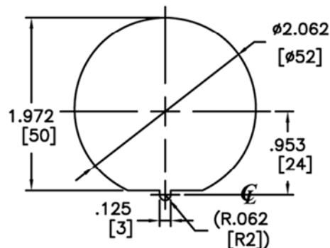
Размеры отверстия для монтажа
